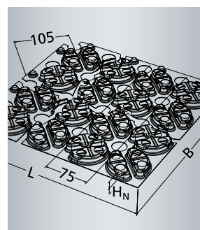
Dimensioni di ingombro del pannello per ristrutturazioni con posa a umido
