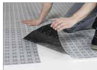
Sovrapposizione minima di 10 cm sul bordo trasversale
