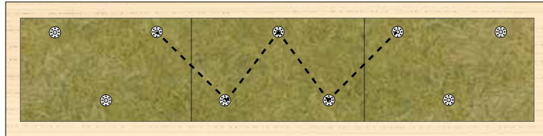
Configurazione REDArt tassello per legno + REDArt Collante DS Per pannello Frontrock Max Plus
