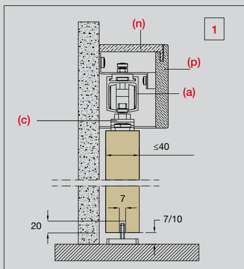
A) Installazione a parete senza zoccolino, per pannelli con spessore (SP) ≤ 40 mm. Installation without skirting board, for door panels of (SP) ≤ 40 mm thick.
