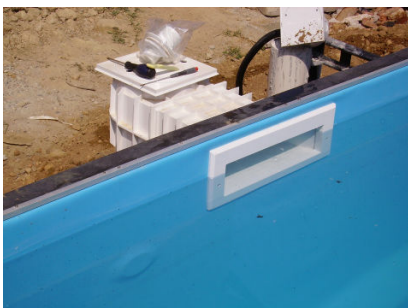
Fase 4: Installazione tubazioni. Si nota il particolare delle controventature ancorate con cemento.
