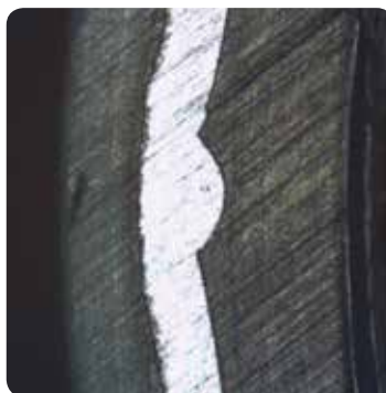
Alluminio saldato di testa (attuale tecnologia)
