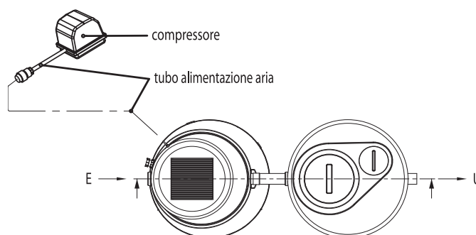
SUPERquattro - Impianto a Fanghi Attivi con filtro percolatore anaerobico
