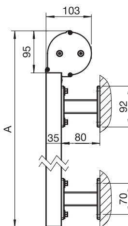
Tessuto arrotolato all'esterno
