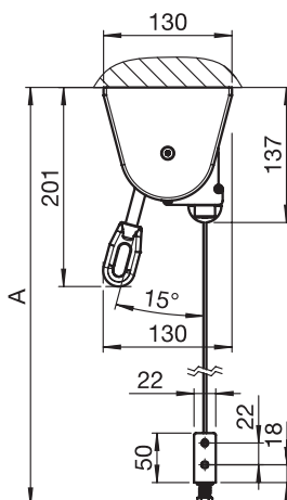
Montaggio a soffitto / in luce
