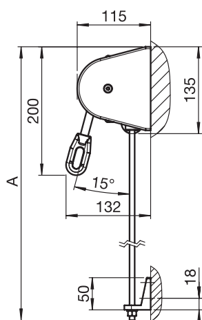
Montaggio a parete
