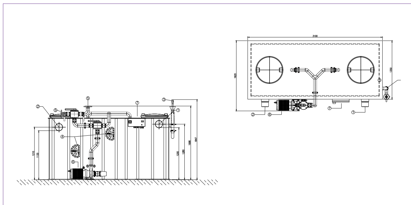
Separatore dei grassi EasyClean NS 15
