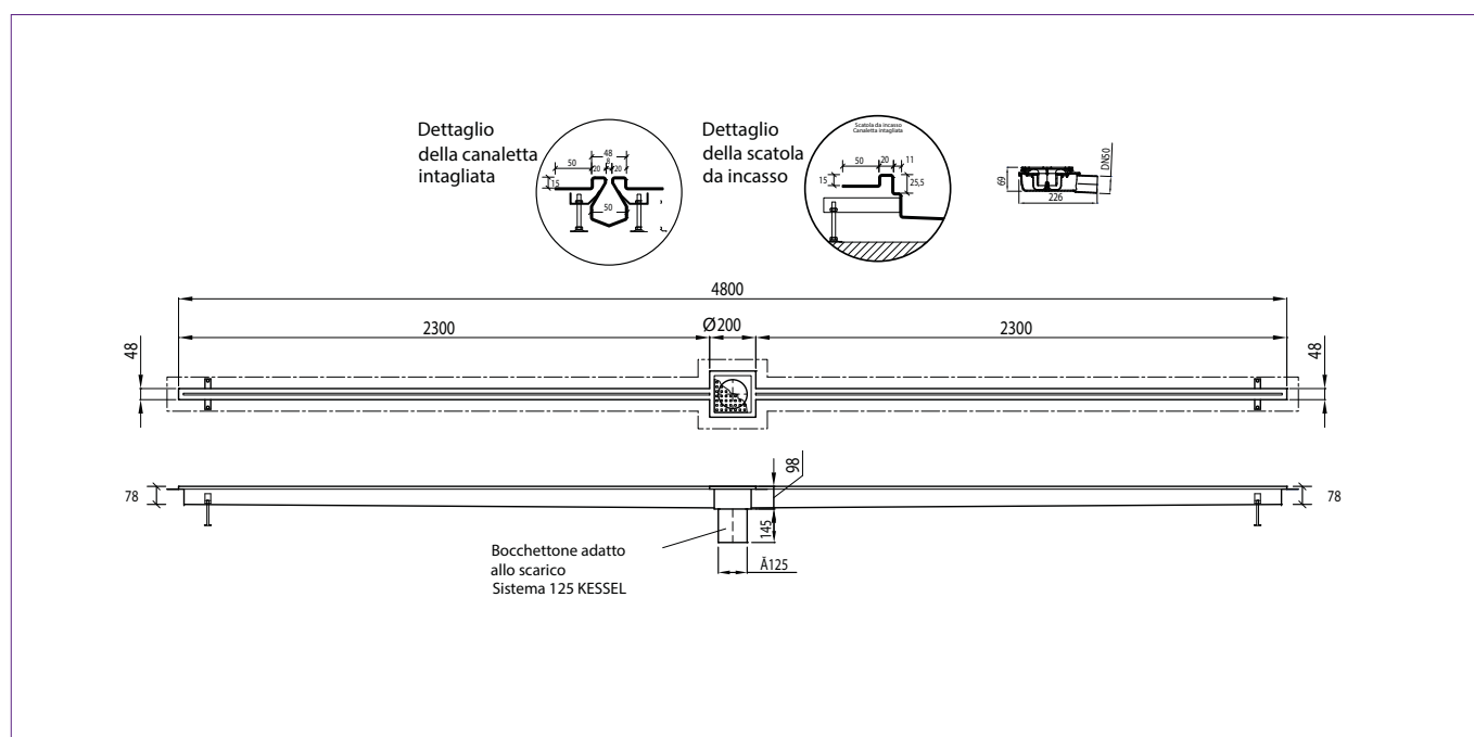
Canaletta intagliata Ferrox Sistema 125
