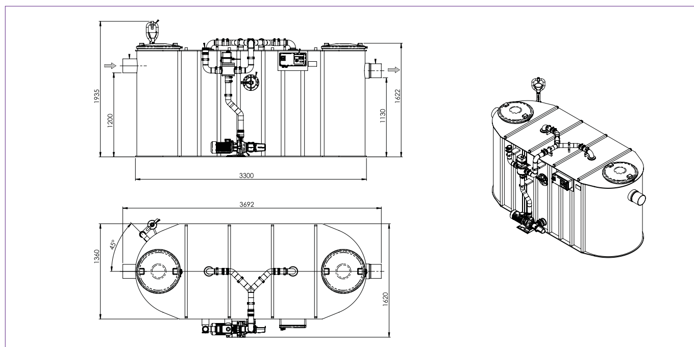
Separatore dei grassi EasyClean NS 15 Auto Mix & Pump
