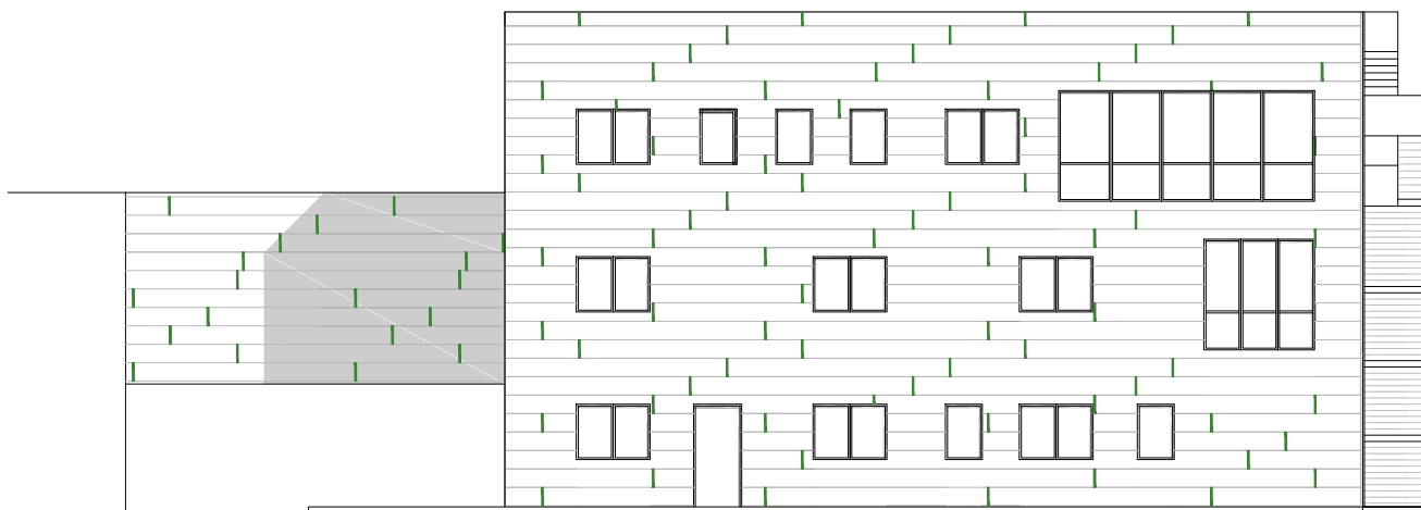
Prospetto Sud South elevation
