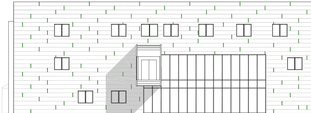
Prospetto Ovest West elevation
