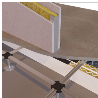
Parete Flessibile
