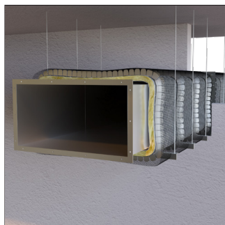
Condotte d'aria orizzontali
