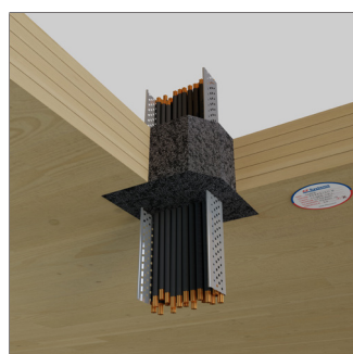
Solaio Xlam
