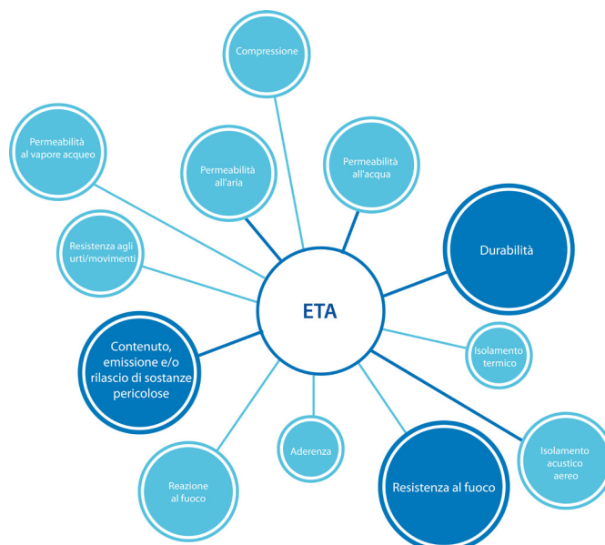
Figura 12 | Le performance certificabili secondo la EAD 350454-00-1106
