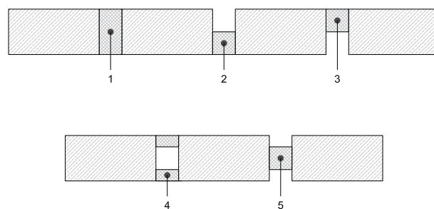
Figura 11 | Posizione delle protezioni antifluo e applicabilità in cantiere
