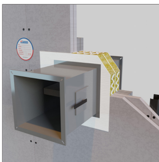
Setto Autoportante
