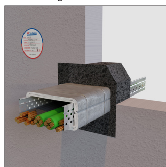
Parete Rigida
