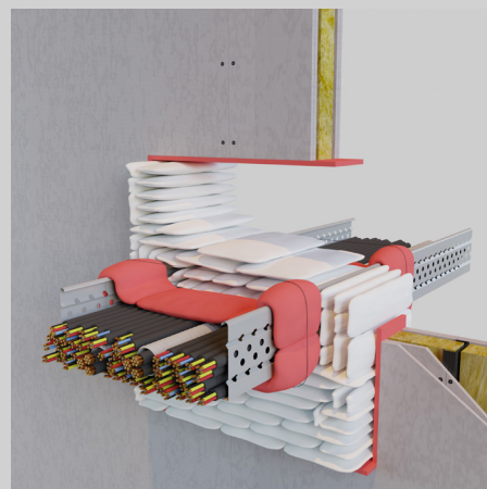
Figura 4c | Profondità di sigillatura 600 mm
