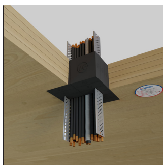
Solaio Xlam
