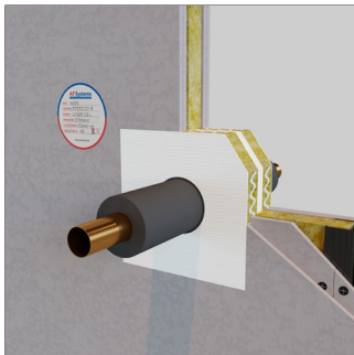
Parete Flessibile
