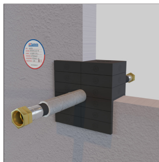
Parete Rigida
