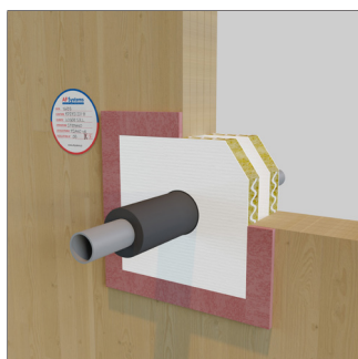
Parete Xlam
