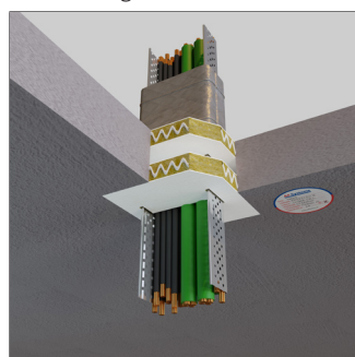
Solaio Rigido
