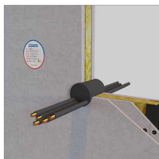
Parete Flessibile
