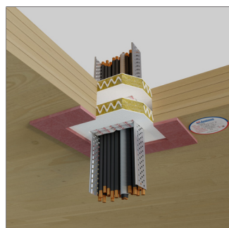
Solaio Xlam
