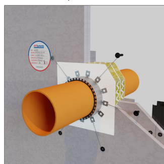
Setto Autoportante
