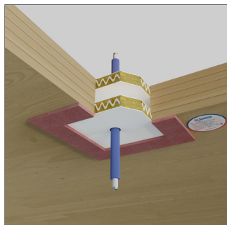
Solaio Xlam
