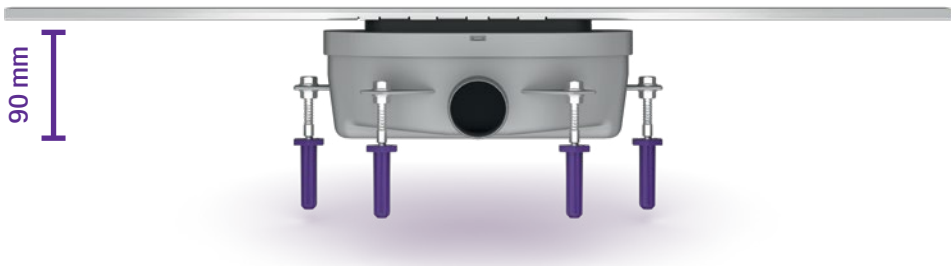
Profondità di installazione di 90 mm con chiusura antiodore di 50 mm
