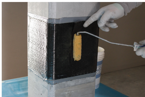
Fase 6: Impregnazione con FASSA EPOXY 200
