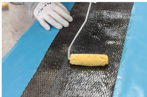
Fase 3: Pre-impregnazione con FASSA EPOXY 200
