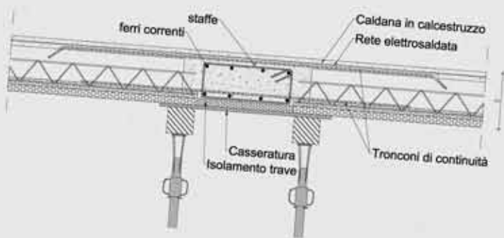
Particolare appoggio su trave a spessore
