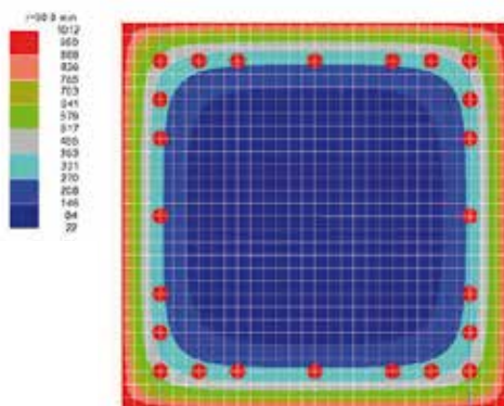
Andamento della temperatura in un pilastro in cemento armato
