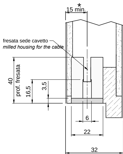
Sez. F-F
