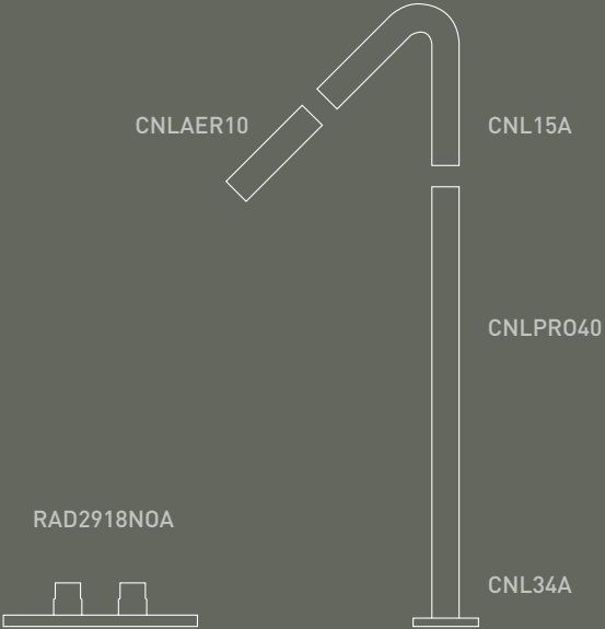
CNLAER10 Aeratore | Aerator | Mousseur | Lufsprudler | Aireador CNL15A Bocca Appoggio | Deck mtd. Spout | Bec sur Meuble | Auslauf | Caño sobre Repisa CNLPRO40 Prolunga | Extension | Rallonge | Verlängerung | Alargo RAD2918N0A Rubinetti Appoggio | Deck mtd. Valves | Mélangeur sur Meuble | Stand Montage Batterie | Bimando sobre Repisa CNL34A Raccordo da Appoggio | Deck Adaptor | Raccord | Adapter | Conexion
