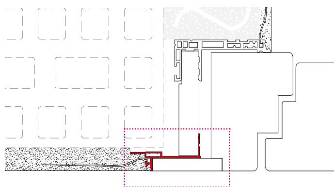
con coprifilo ADDOSSATO AL MURO
