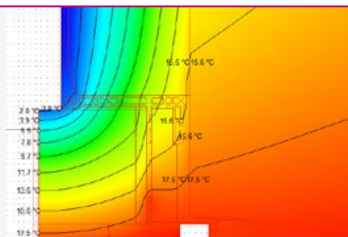
Termografia soluzione con coprifilo distanziato dal muro
