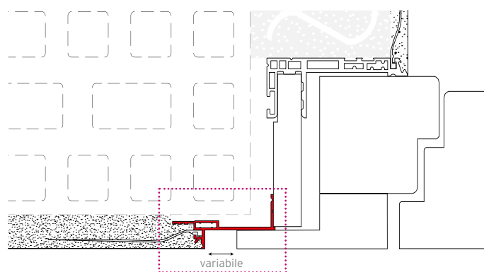
con coprifilo DISTANZIATO DAL MURO
