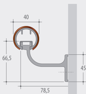
Mensola in alluminio anodizzato ECO
