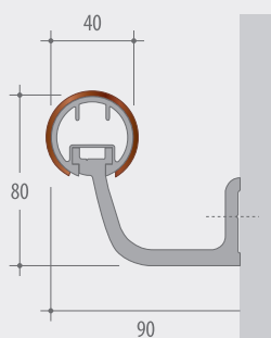
Mensola in alluminio anodizzato
