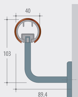
Mensola in acciaio inox
