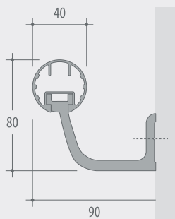
Mensola in alluminio anodizzato
