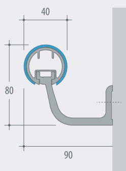
Mensola in alluminio anodizzato
