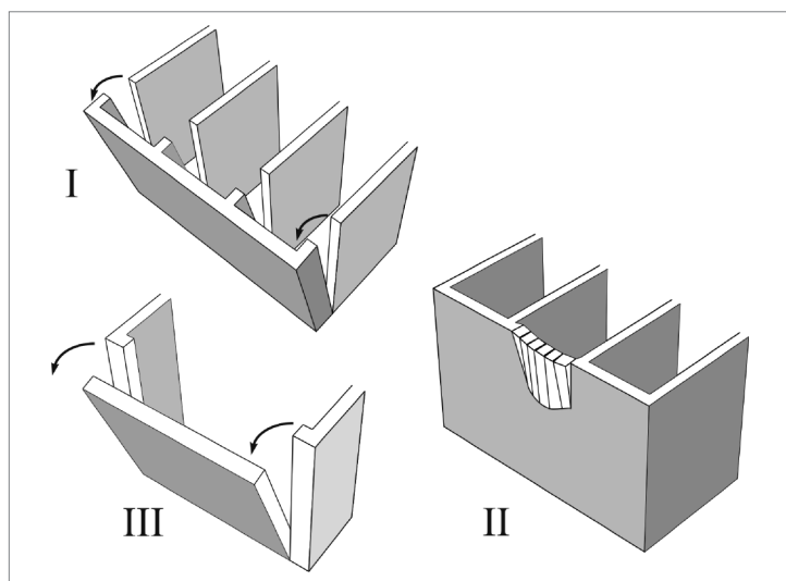
Fig. 1. Modi di rottura: I, II, III
