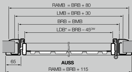
Sezione orizzontale
