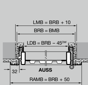
Sezione orizzontale
