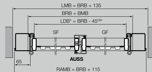
Sezione orizzontale
