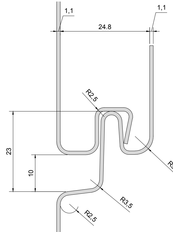
DETTAGLIO RILLATURA
