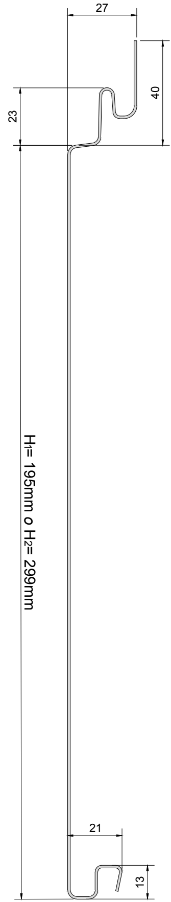
SEZIONE 1 ALU-SKIN LISCIA
