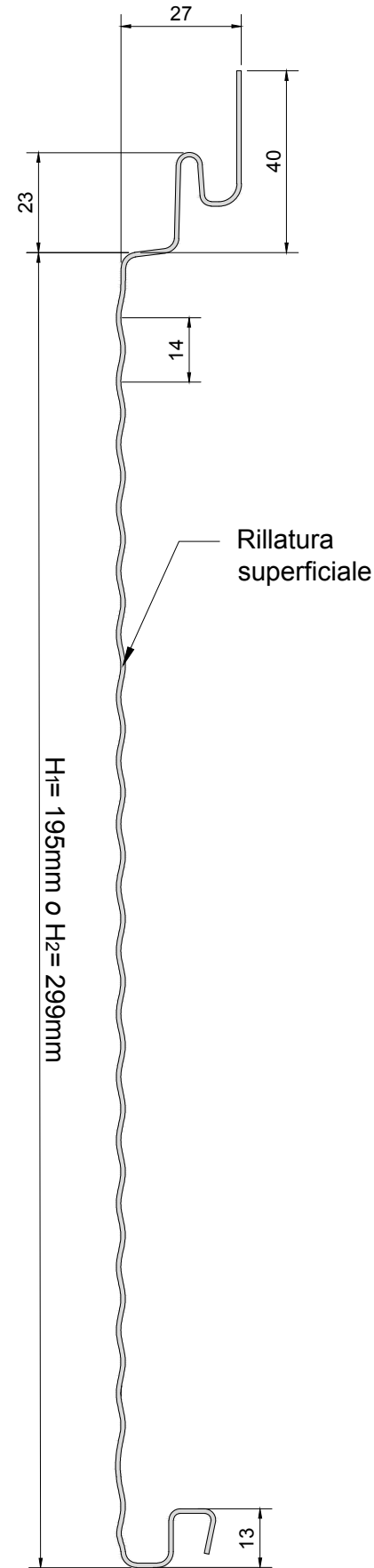
SEZIONE 2 ALU-SKIN RILLATA
