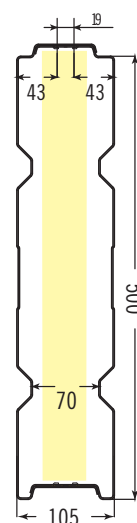
SEZIONE PANNELLO PANEL SECTION
