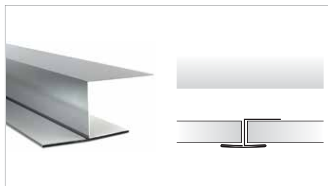
Giunzione intermedia PL02 Junction flashing PL02
