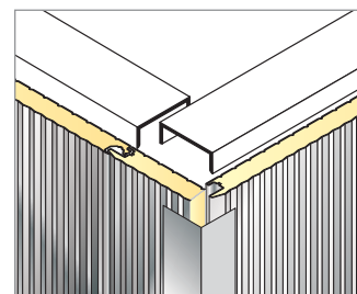
Sezione tipo Type section
