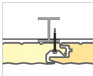
Fissaggio su metallo Fixing on metal
