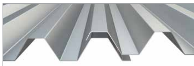
Sovrapposizione laterale di una greca con piedino di appoggio Lateral overlapping of a corrugation with support
