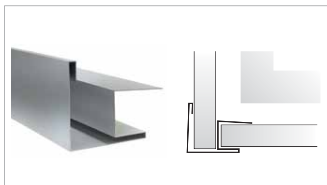
Angolo esterno PL03 External corner PL03
