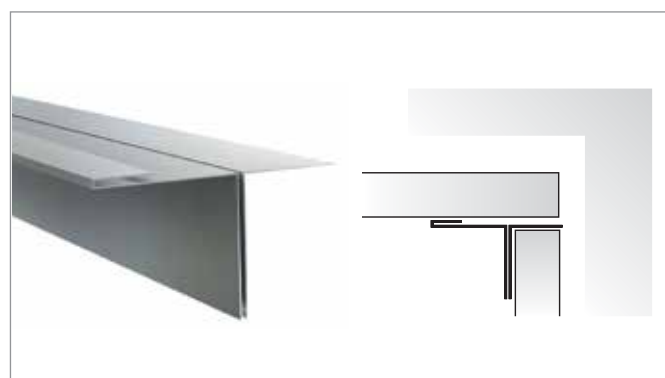
Angolo interno PL04 Internal corner PL04
