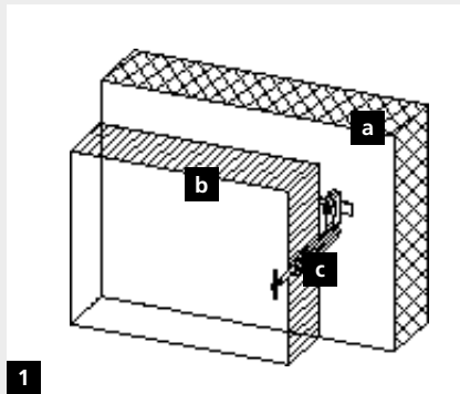
1 Sistema di ancoraggio: mensola e ancoraggio
