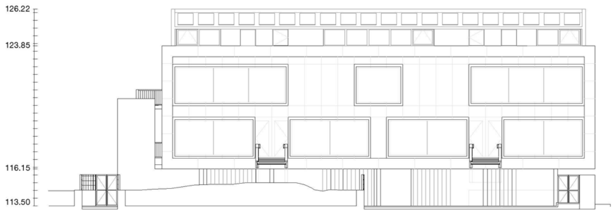
Prospetto sud
