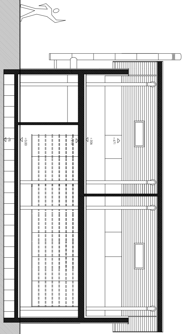
SEZIONE D-D
