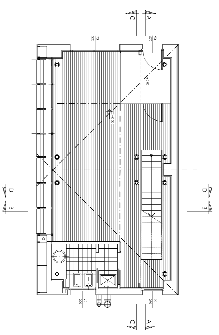
PIANTA PIANO TERRA-RAPPORTI PROPORZIONALI
