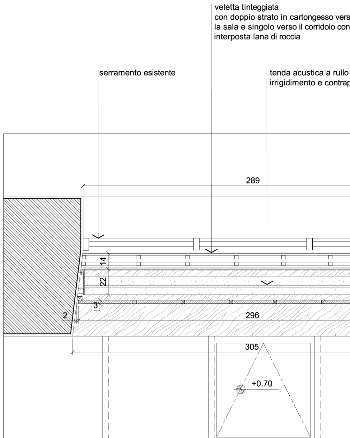
DETTAGLIO 1 SEZIONE A-A - scala 1:20
