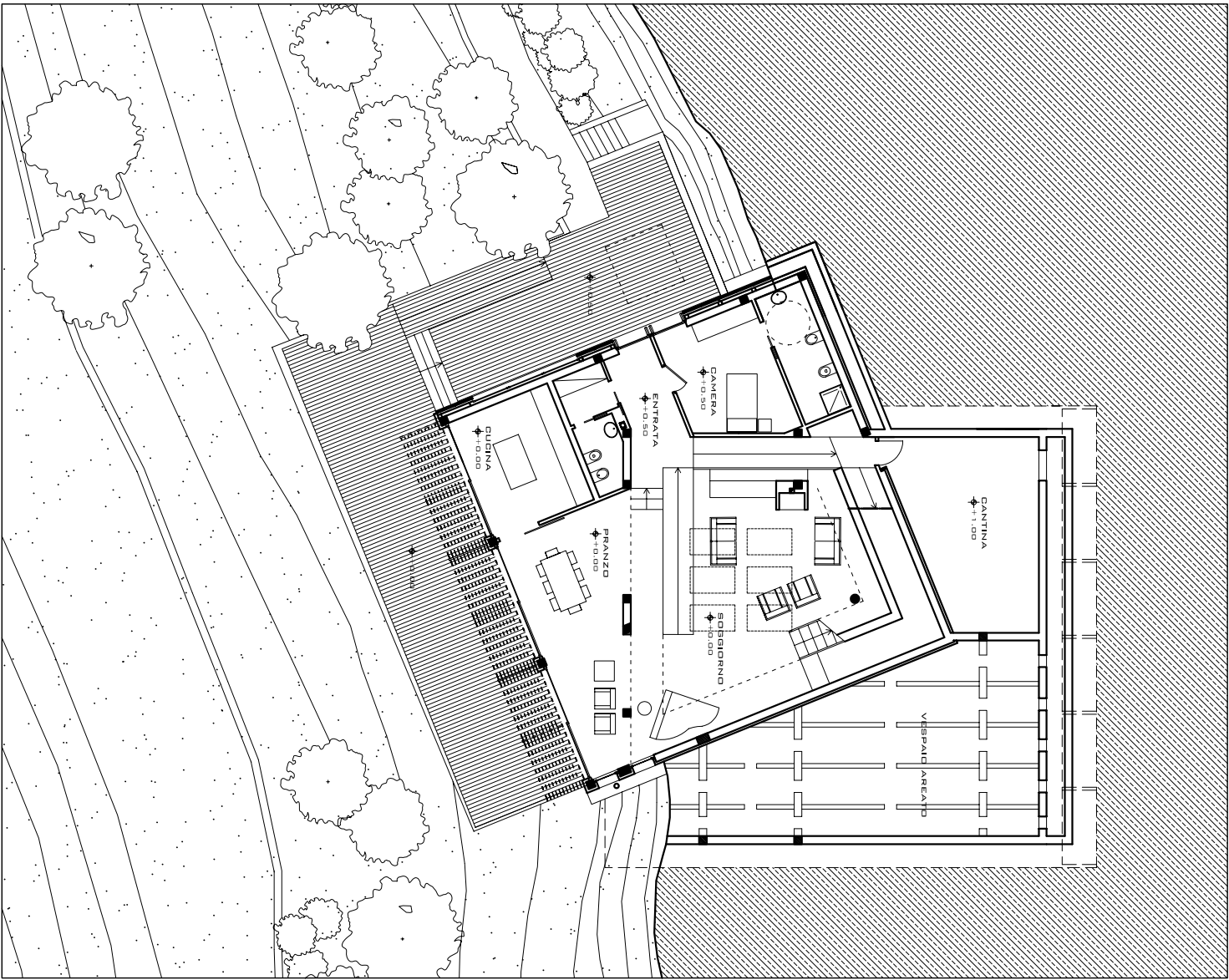
LIVELLO + 0.50
