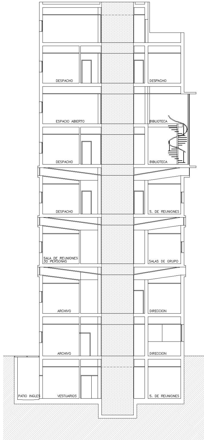
SECCION B-B
