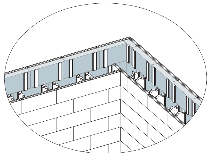
Particolare tavella per il contenimento solaio
