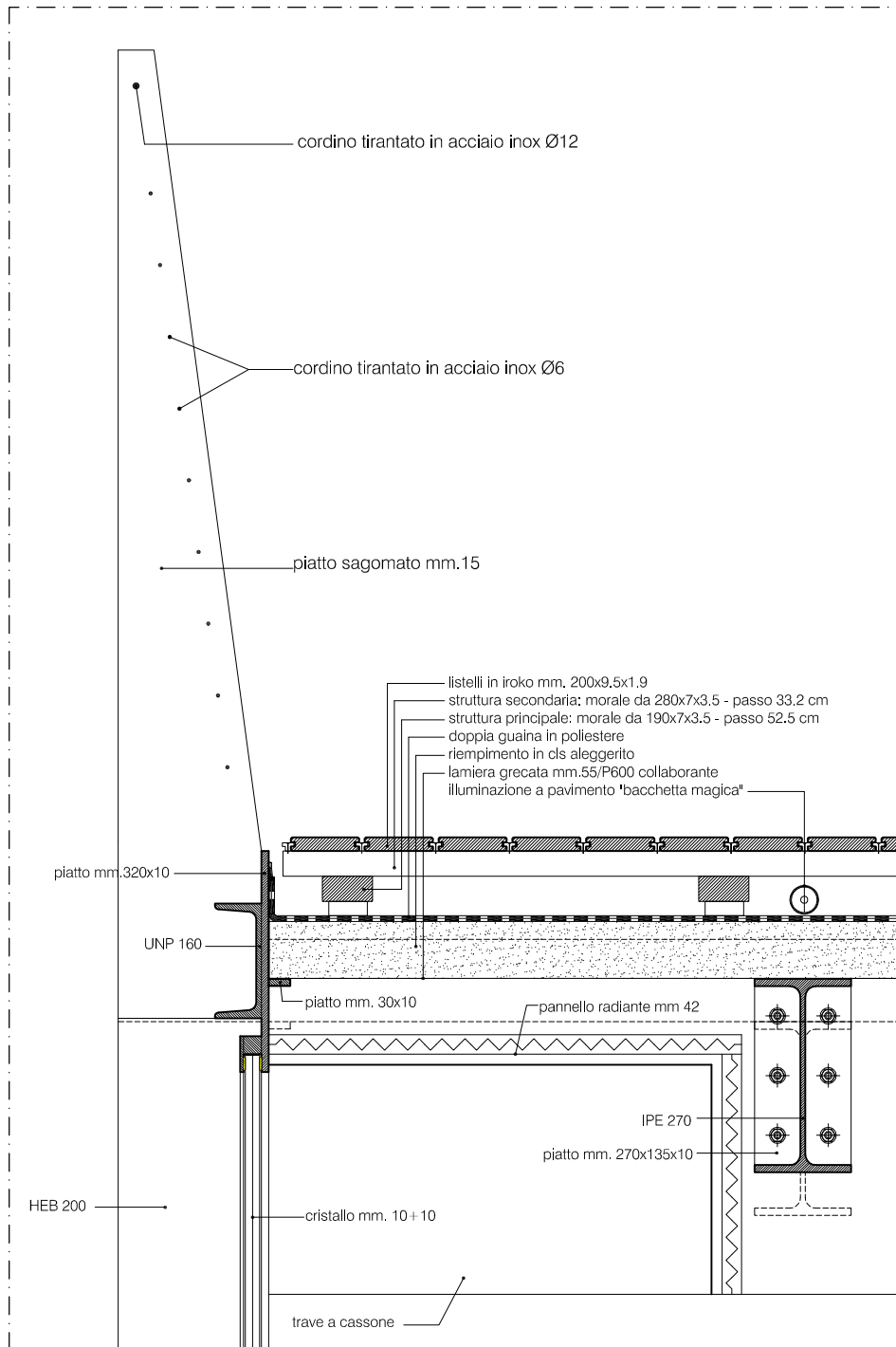
01 - DETTAGLIO SEZIONE PASSERELLA
