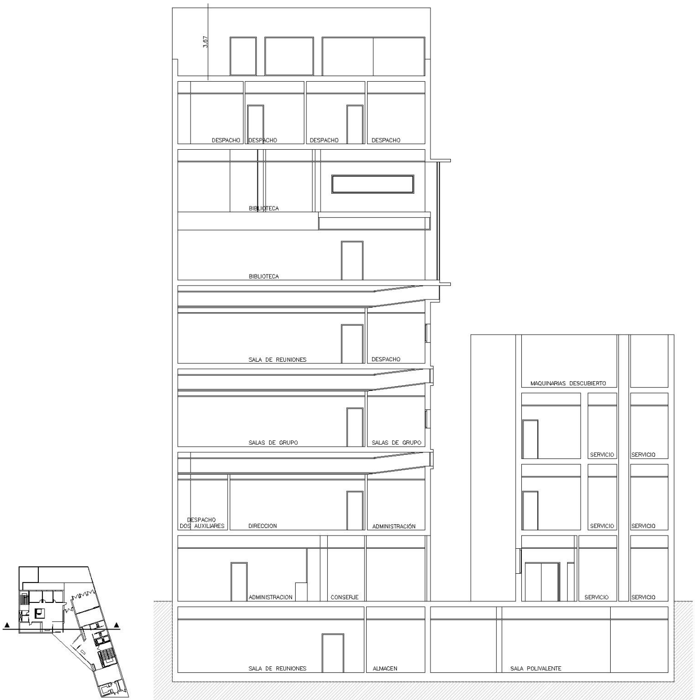
SECCION A-A
