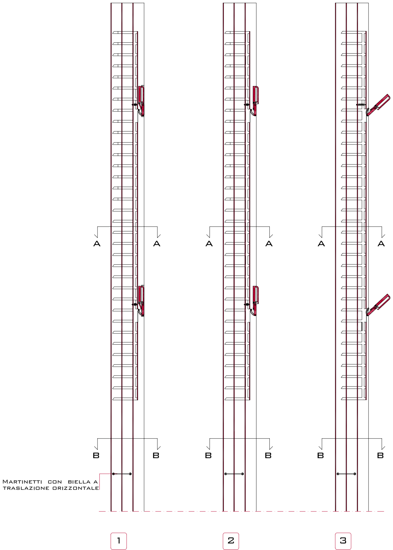
SEZIONE ESPLOSA DEL MONTATE E FASI DI SBLOCCAGGIO DEI PANNELLI
