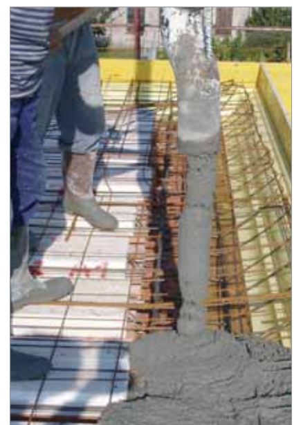
Fasi del getto
