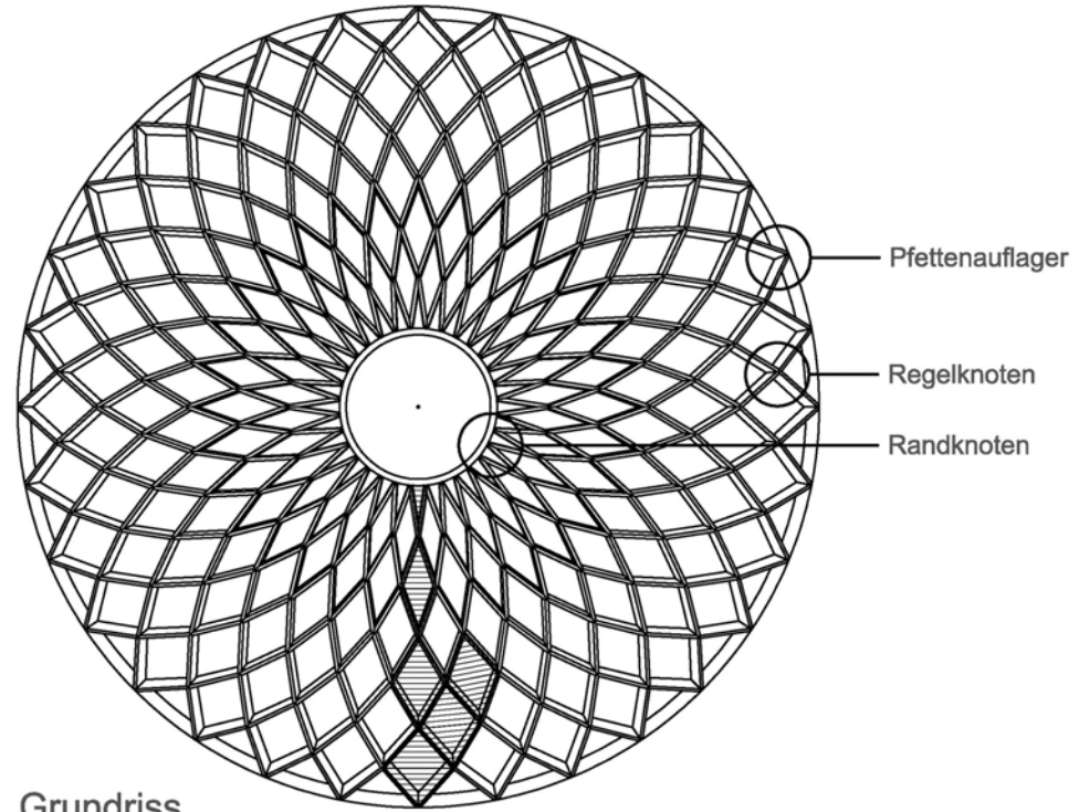
Grundriss
