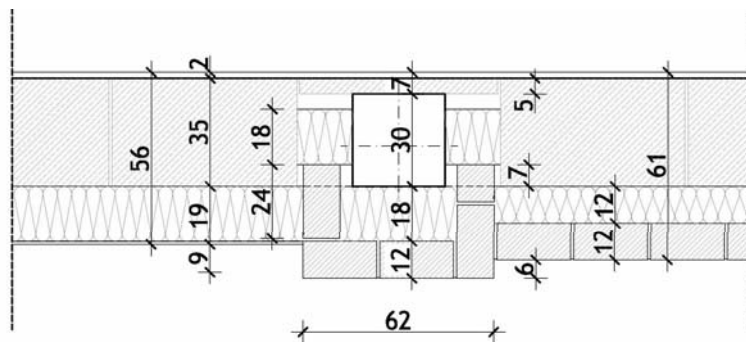
SEZIONE ORIZZONTALE MURATURA IN MATTONI FACCIA A VISTA
