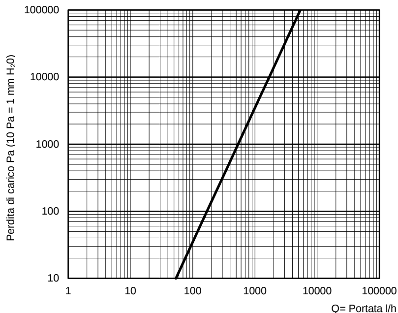
Diagramma perdite di carico
