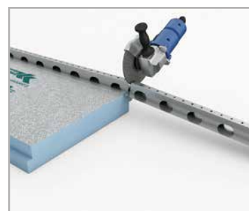
Taglio del correntino
