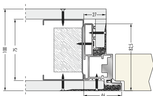
Telaio su parete in cartongesso con una lastra Spessore parete finita 100 mm
