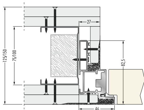
Telaio su parete in cartongesso con due lastre Spessore parete finita 125/150 mm
