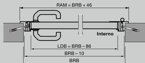
Porta pedonale laterale con telaio ad angolo in alluminio, profilo tipo 3 Battuta esterna
