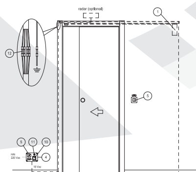
Esempio installazione su esistente Example of installation on existing frame
