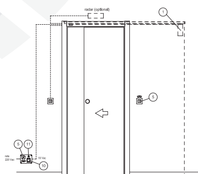
Esempio installazione sul nuovo Example of installation on new frame
