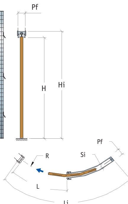
apertura DESTRA RIGHT opening
