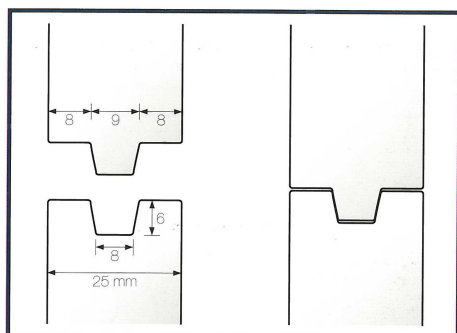
PARTICOLARE INCASTRO
