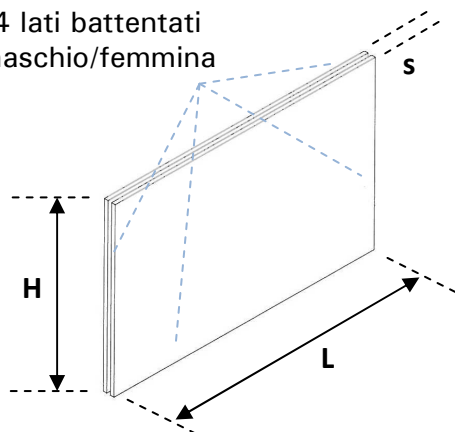
PARTICOLARE INCASTRO
