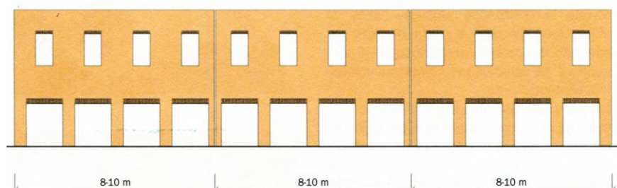
I DUE FONDAMENTALI TIPI DI GIUNTO DI DILATAZIONE VERTICALE PER LE MURATURE IN MATTONI FACCIA A VISTA SONO: RETTILINEO E DENTATO
