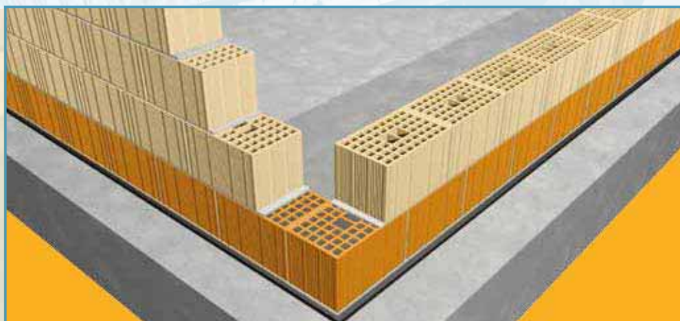
Nodo costruttivo: piede della muratura
