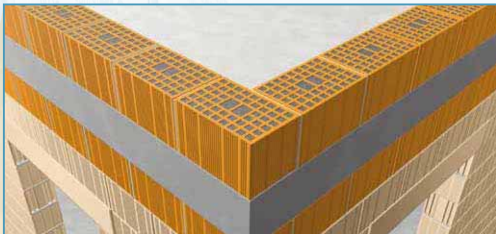
Nodo costruttivo: solaio
