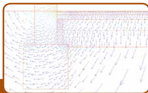
Direzione del flusso termico.
