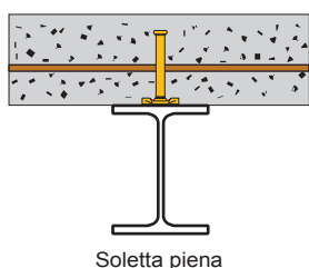
Soletta piena
