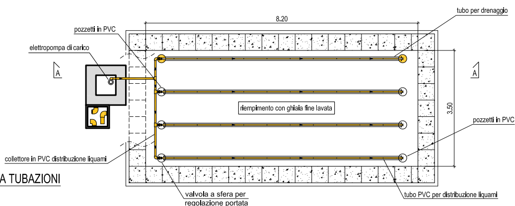
PIANTA FONDO BACINO DI DEPURAZIONE
