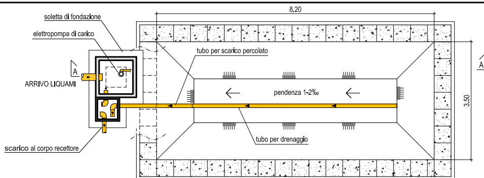
PIANTA FONDO BACINO DI DEPURAZIONE
